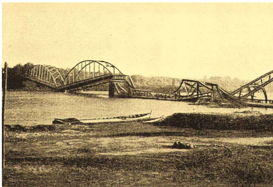
Most w Zegrzu wysadzony przez polskich saperów w nocy z 6 na 7 września 1939 r. („Denkschrift über die polnische Landesbefestigung”, Berlin 1941, s. 70)
